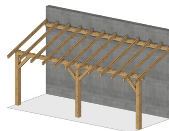
Auvent
