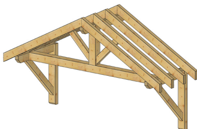
Marquise 2 pans
